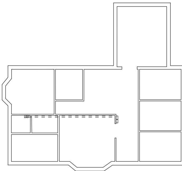
Рис. 5.1.2 План стен и перегородок.
