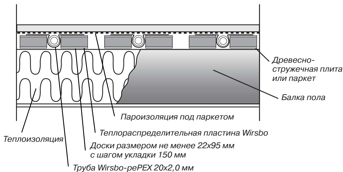
Рис. 3.5.1 Поперечное сечение петли трубы с теплопроводящими пластинами.
