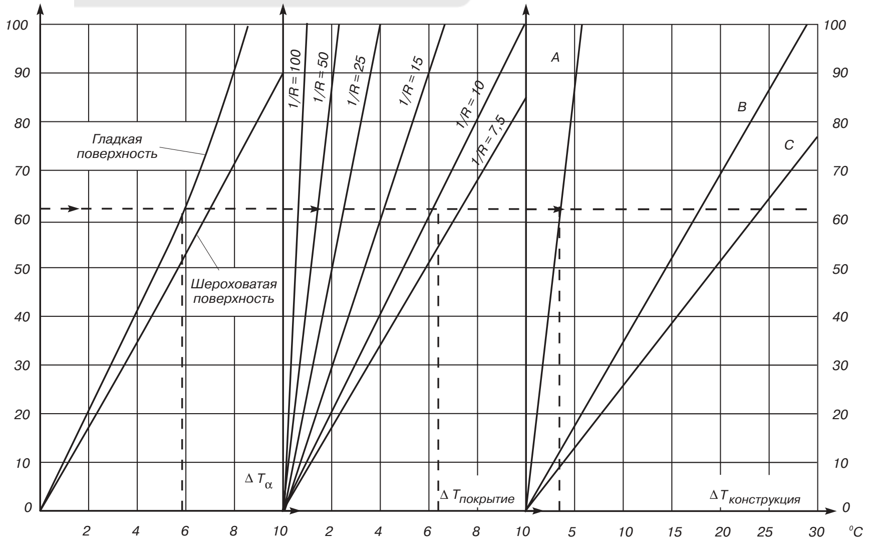
Диаграмма 8.2.1 Средняя температура воды/потери тепла.
